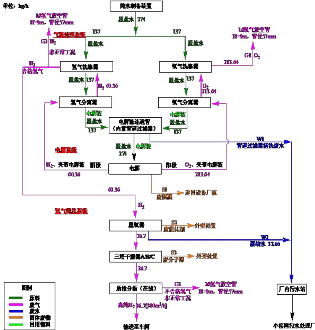
图 3-9 单套水电解制氢及纯化装置小时物料平衡图
