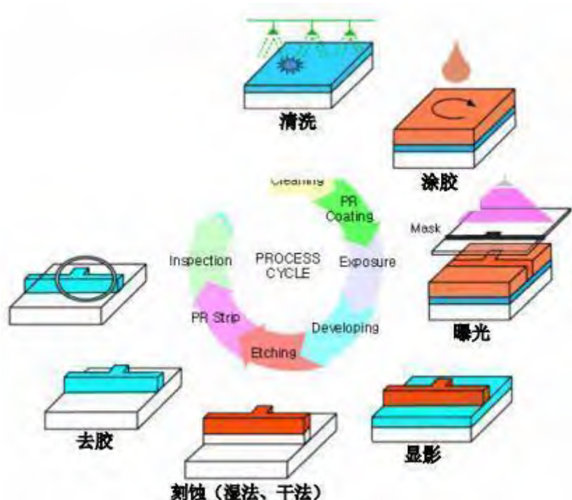
图 2-10 光刻过程示意图
