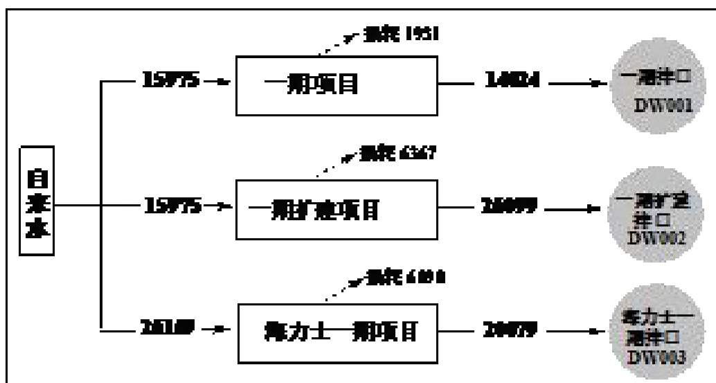
图 2-2 现有工程水平衡图 (m³/d)
