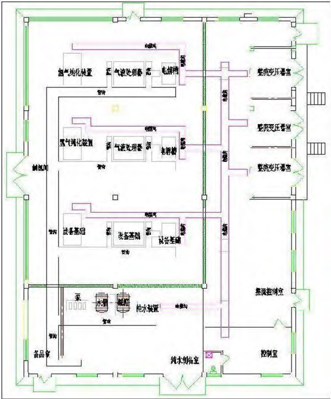
图 2-23 扩建前制氢站车间平面布置图（联华精密气体站）
