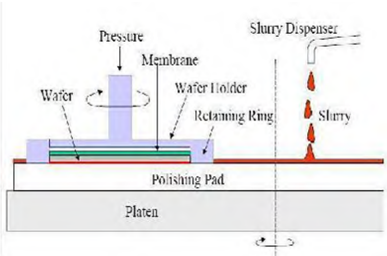
图 2-13 化学机械研磨工艺示意图
