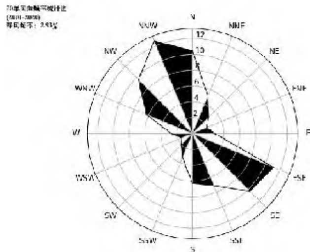
图 4-1 大连风向玫瑰图（静风频率 1.3 %）
